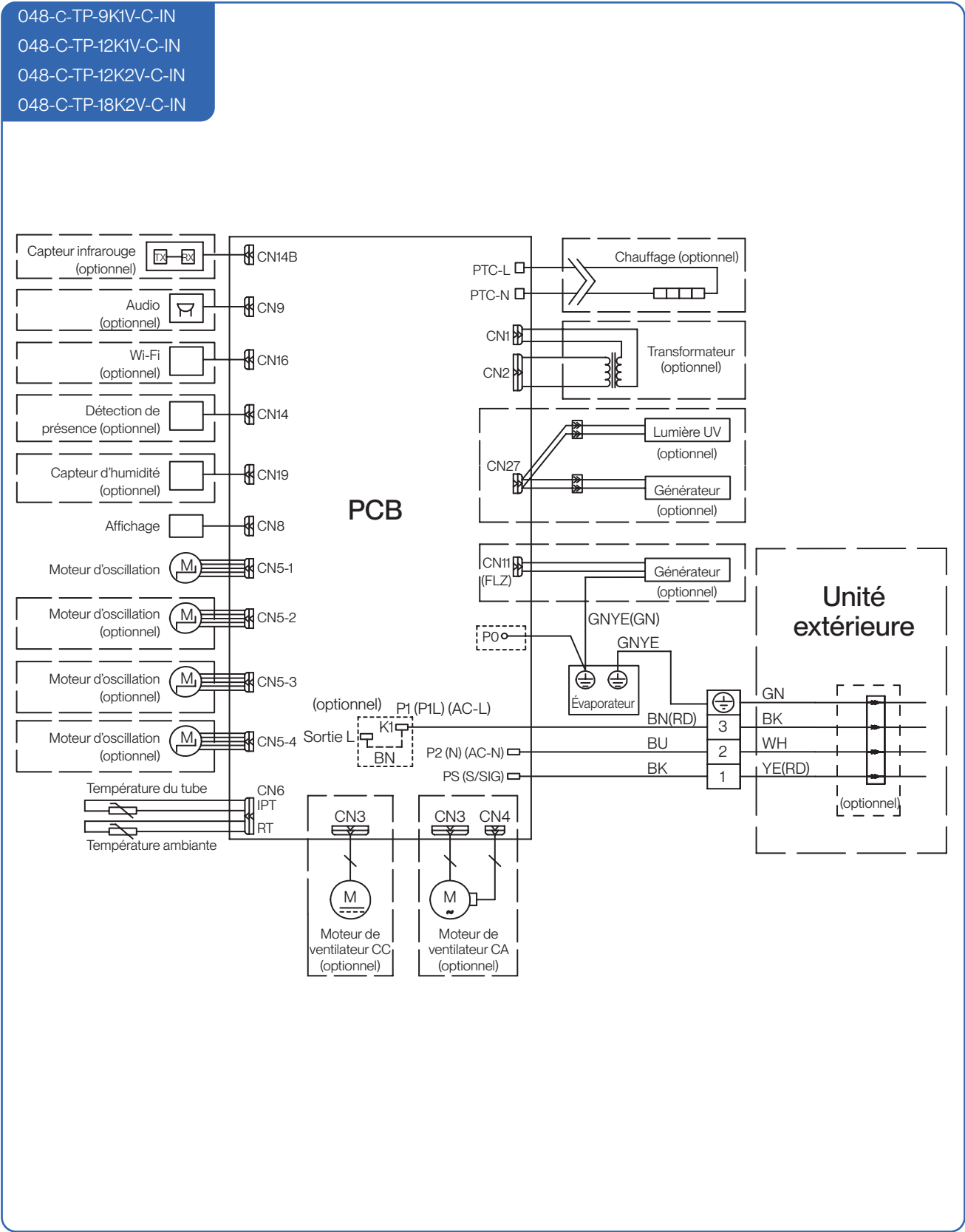
Schéma électrique de l'unité intérieure
